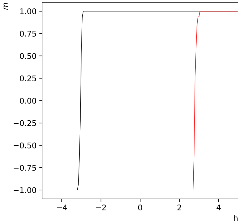
Hystérésis de l'aimantation réseau de taille L=8 - h=5 à T=0.5
