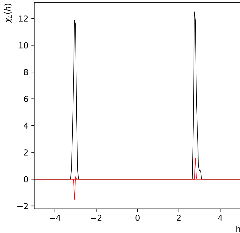
\chi_L(h) réseau de taille L=8 à T=0.5
